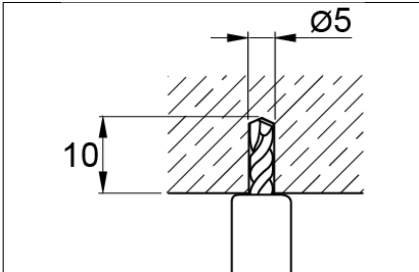
Vorbohren mit Hilti TX-C-5/10B Bohrer
