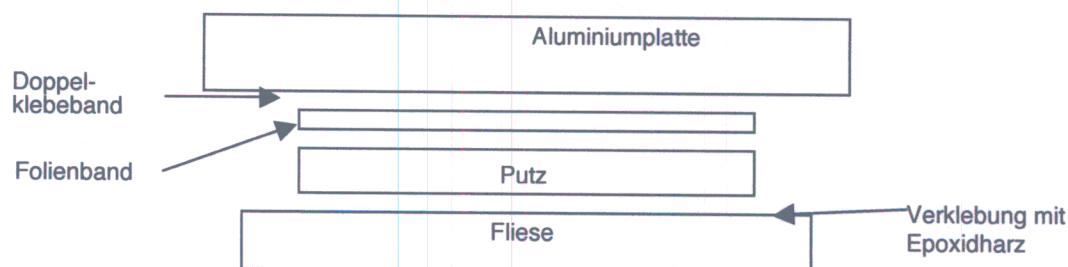
Bild 1: Probekörperaufbau, schematisch
